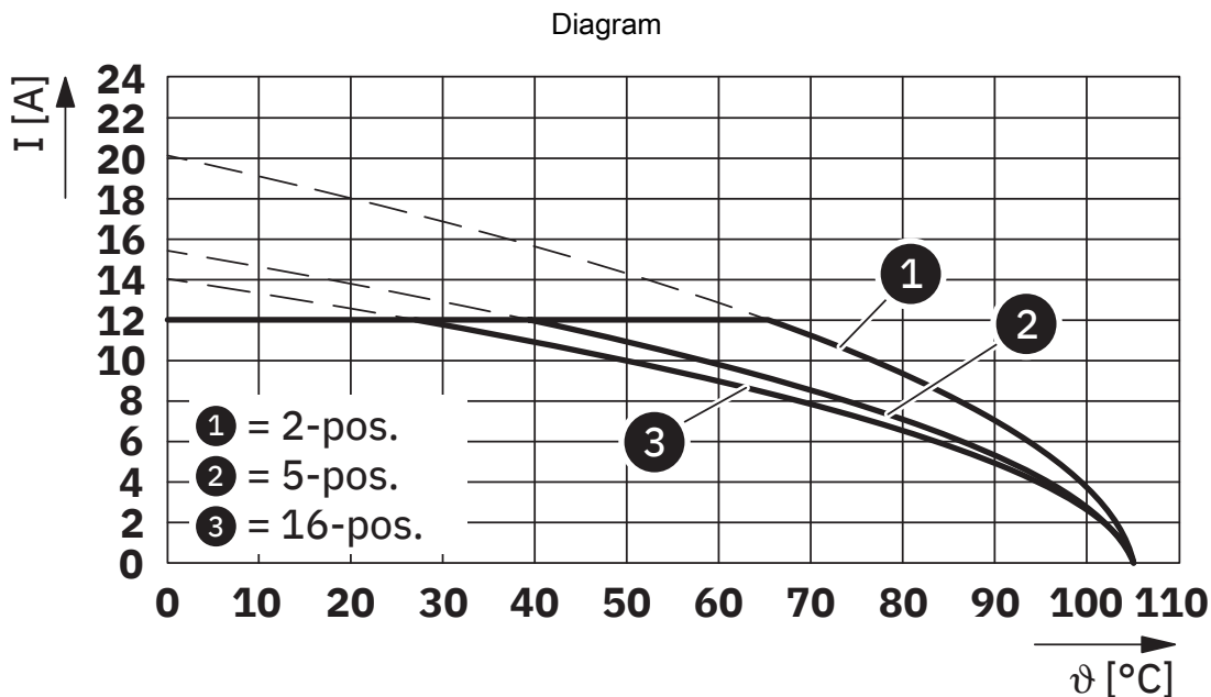
Type: FKC 2,5/...-STF-5,08 AU with MSTBV 2,5/...-GF-5,08 AU
