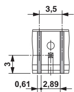
外形寸法
