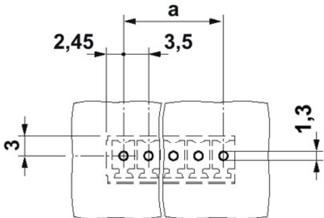
穴あけ加工図
