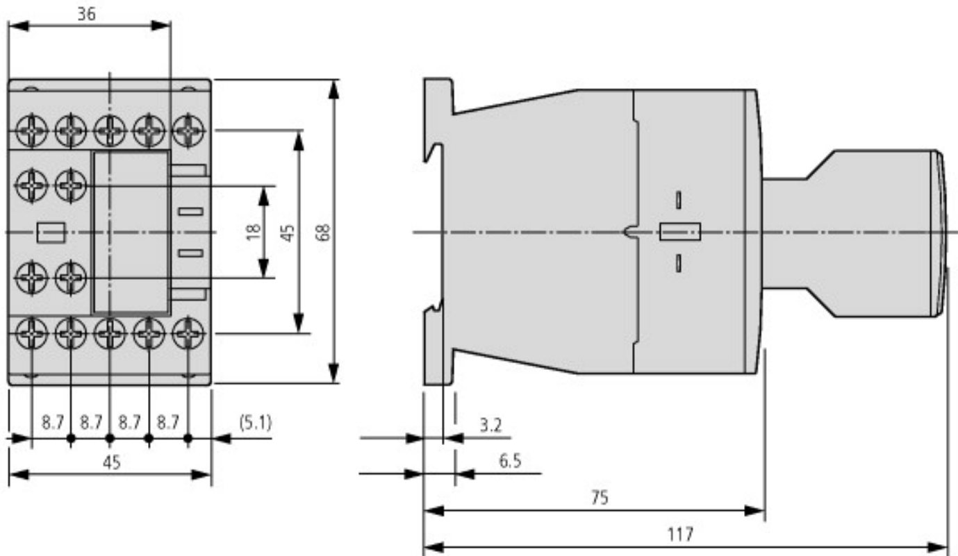
Contacteur with auxiliary contact module
