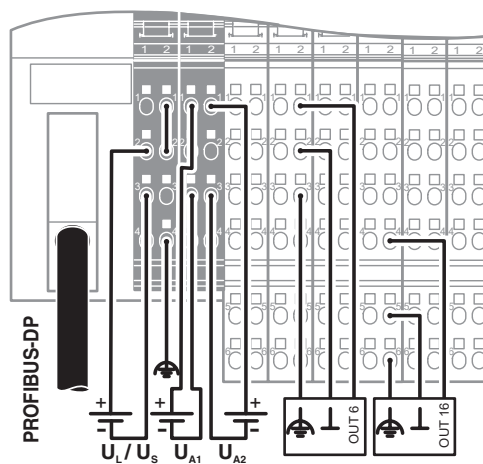
DI 16 DO 16
