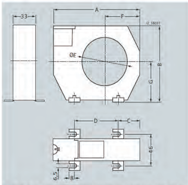
剩余电流互感器, 5SV8 702-0KK, 5SV8 703-0KK, 5SV8 704-0KK, 5SV8 705-0KK, 5SV8 706-0KK
