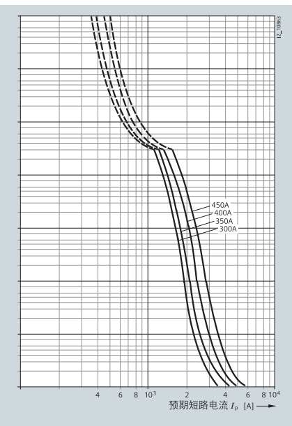
时间—电流特性图
