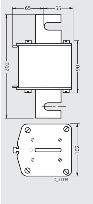
尺码4 (IEC标准)
