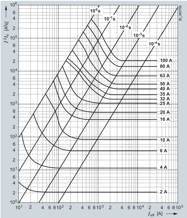
熔化 I^2t 图
