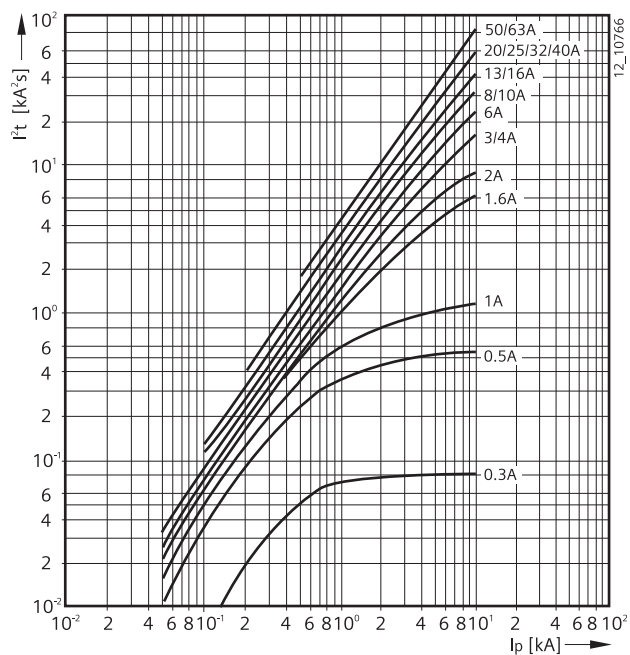
C特性
