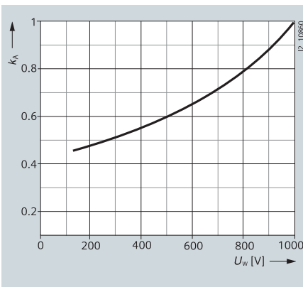
分断I^2t值校正系数
