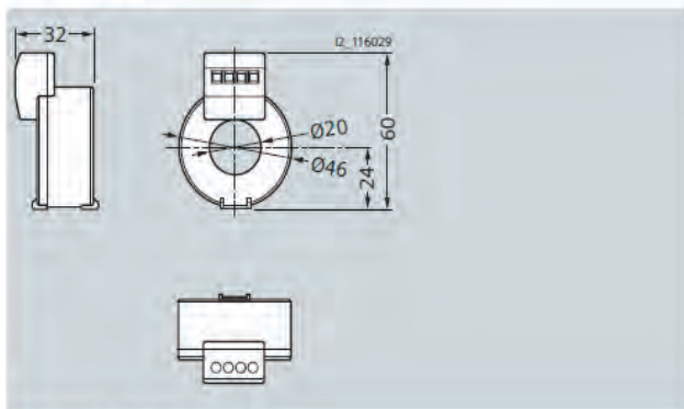
剩余电流互感器, 5SV8 700-0KK
