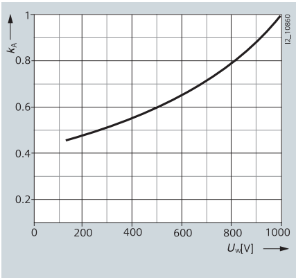
分断I^2t值校正系数
