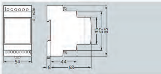
RCM 数字式, 5SV8 001-6KK, 5SV8 200-6KK
