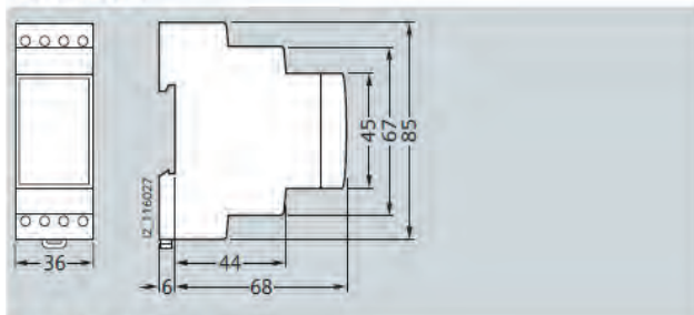
RCM 模拟式, 5SV8 000-6KK
