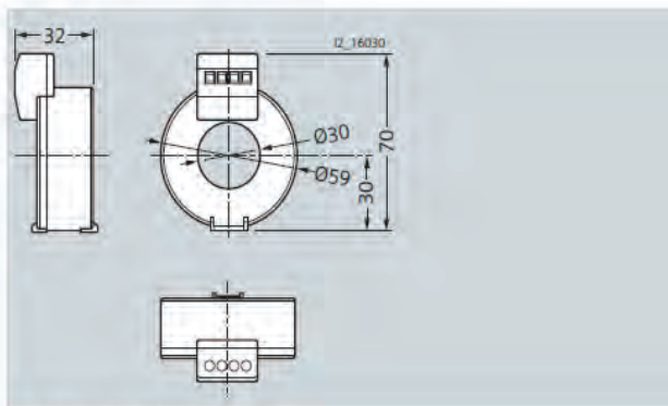
剩余电流互感器, 5SV8 701-0KK
