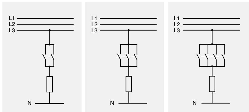
2 poles in //
