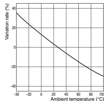
G3NA-2□□B AC input
