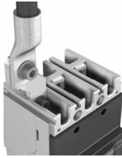
Terminal ES with cable lug
