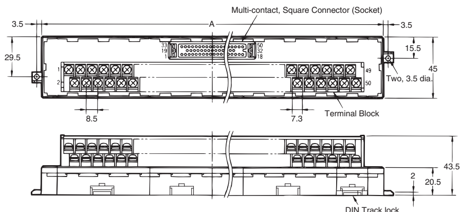
Dimensions
