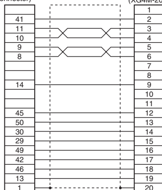
XW2Z-200J-B2
