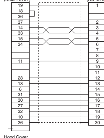
XW2Z-200J-B3
