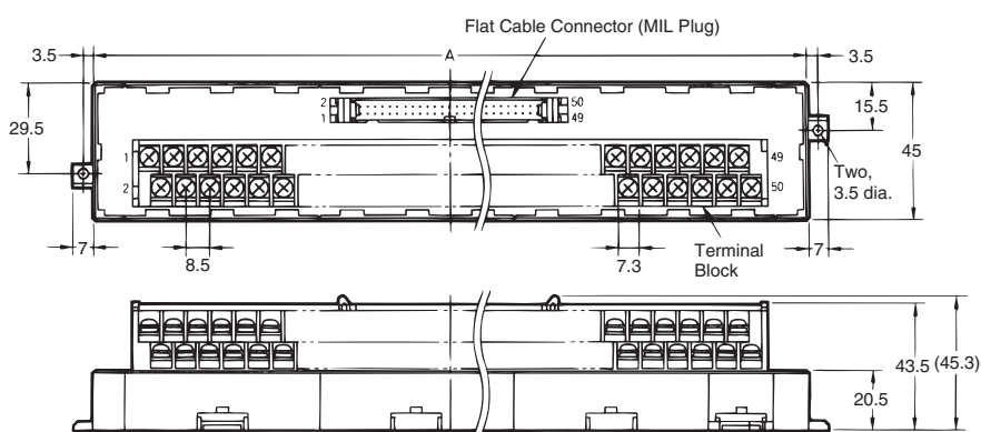
Dimensions
