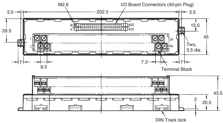
Dimensions
