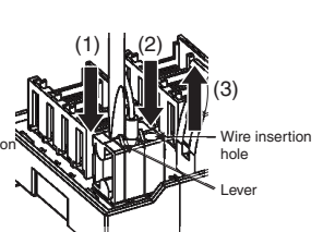
XW2N-202G-IN16
