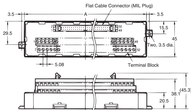
Dimensions
