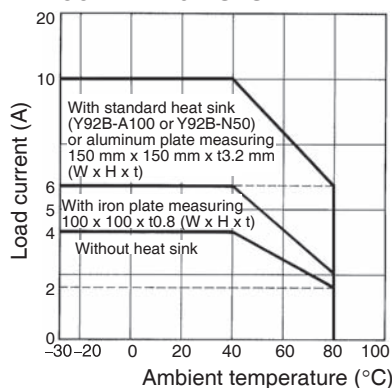
G3NA-D210B-UTU
