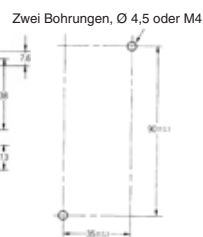
Befestigungsbohrungen
