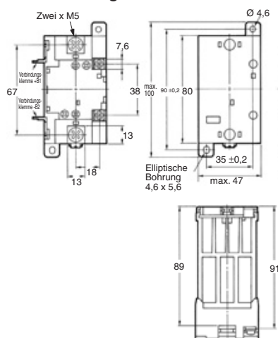
Ohne Klemmen- abdeckung
