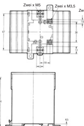
Ohne Klemmen- abdeckung
