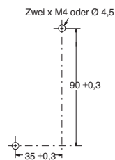
Befestigungsbohrungen
