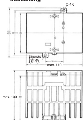
Mit Klemmen- abdeckung
