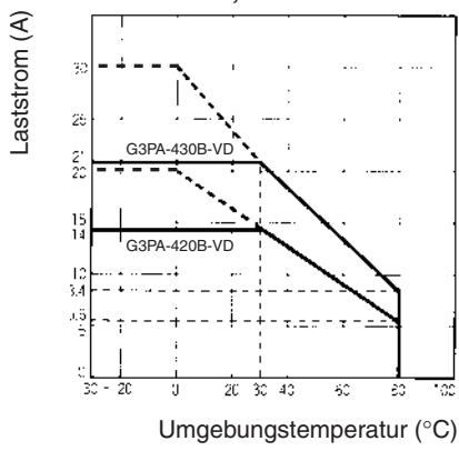
G3PA-420B-VD, G3PA-430B-VD G3PA-420B-VD-2, G3PA-430B-VD-2
