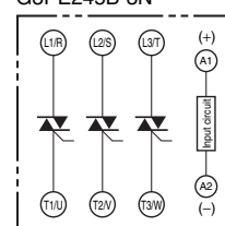
G3PE245B-3N
