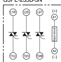
G3PE-235B-3N
