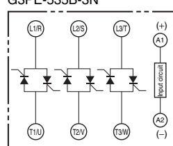
G3PE-535B-3N
