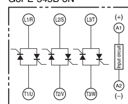
G3PE-545B-3N
