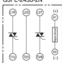
G3PE-245B-2N
