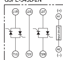
G3PE-545B-2N
