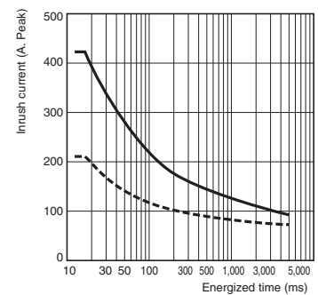
G3PE-535B(L), G3PE-545B(L)
