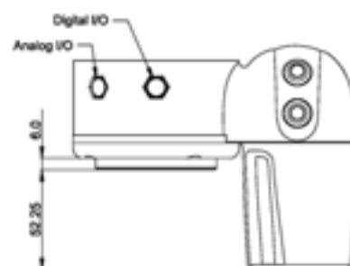
Flange
