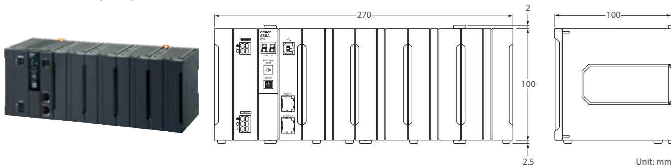
S8BA-24D24D480LF (480 W)
