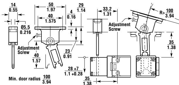
Flexible 1 Actuator
