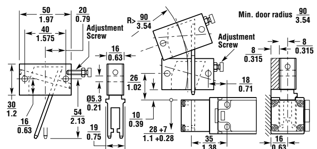
Flexible 2 Actuator
