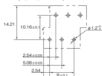
プリント基板加工寸法 (BOTTOM VIEW)
