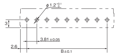
プリント基板加工寸法 (BOTTOM VIEW)
