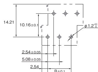
プリント基板加工寸法 (BOTTOM VIEW)
