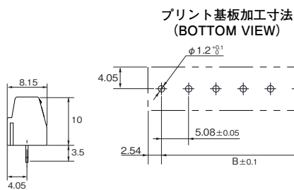
寸法表
