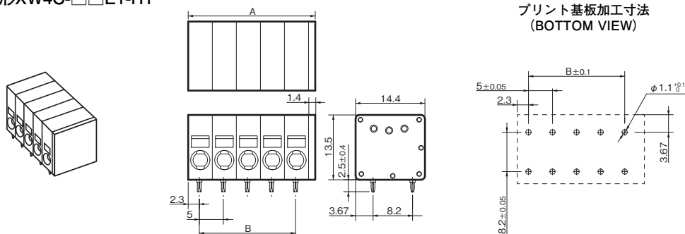
寸法表
