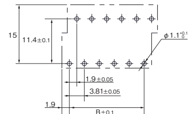
プリント基板加工寸法 (BOTTOM VIEW)
