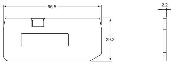
XW5E-P4.0-1.1-2
