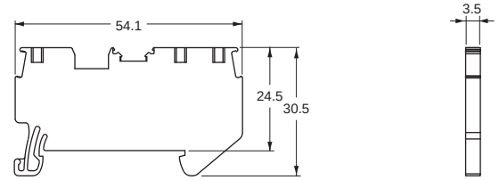
XW5T-P1.5-1.2-1 (BL)/XW5G-P1.5-1.2-1
