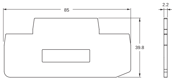
XW5E-P4.0-1.1-2
