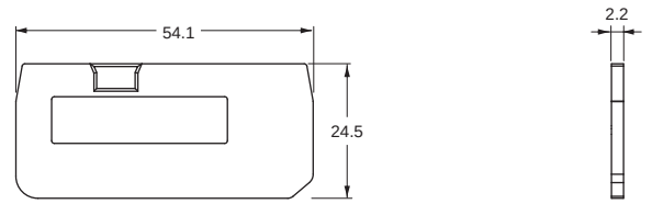
XW5E-P1.5-1.1-2
