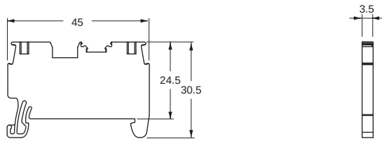
XW5T-P1.5-1.1-1 (BL)/XW5G-P1.5-1.1-1
