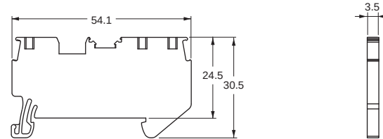
XW5T-P1.5-1.2-1 (BL)/XW5G-P1.5-1.2-1
