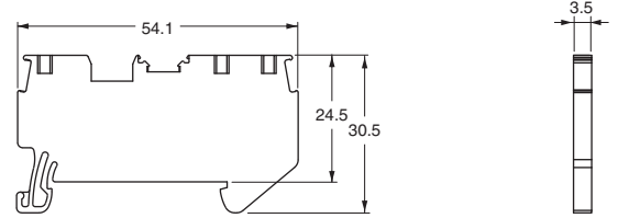
XW5T-P1.5-1.2-1 (BL)/XW5G-P1.5-1.2-1
