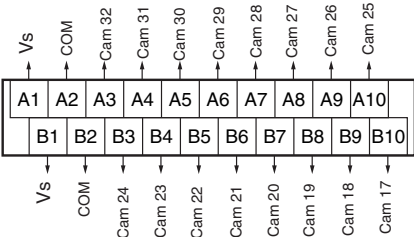
Output Cable 2
