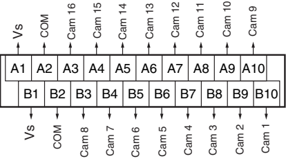
Output Cable 1
